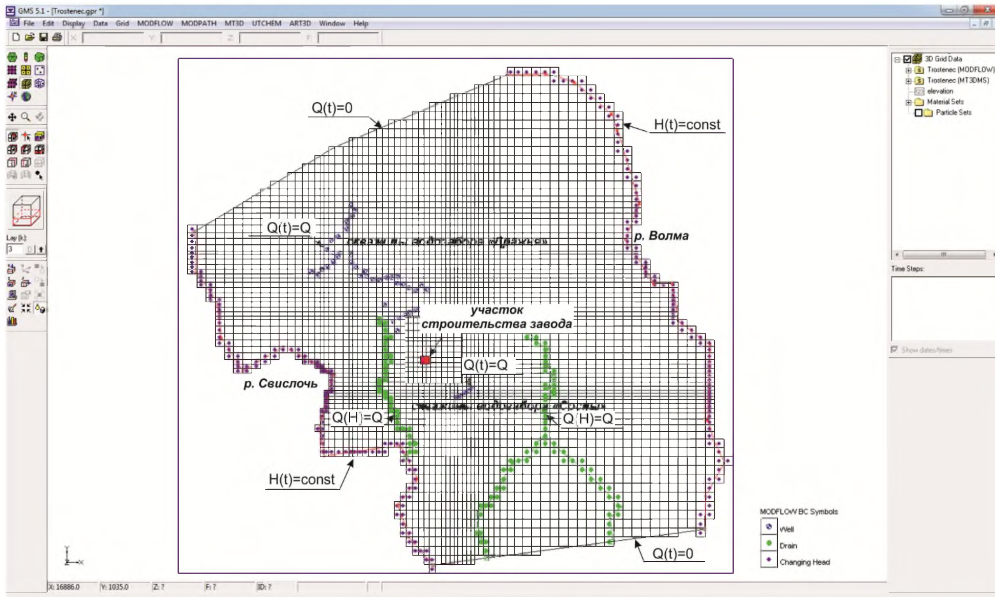
Рисунок 4.1 – Схема геофильтрационной модели в плане
